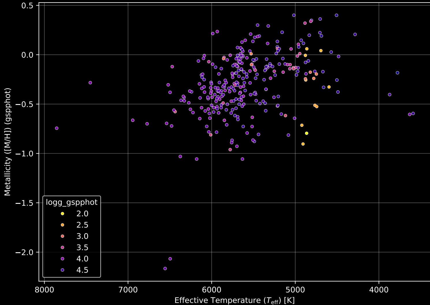
GALAH DR4 Field: [7007] Stellar Population Parameters (n= 307)
