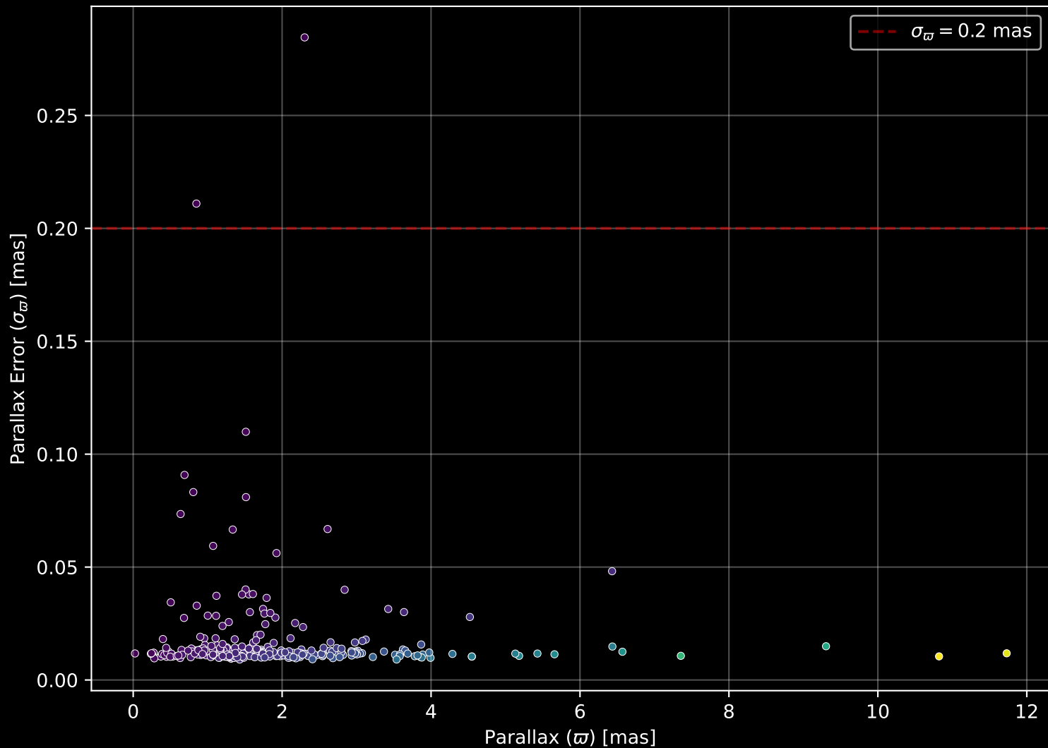
GALAH DR4 Field: [7007] Parallax Quality (n= 307)
