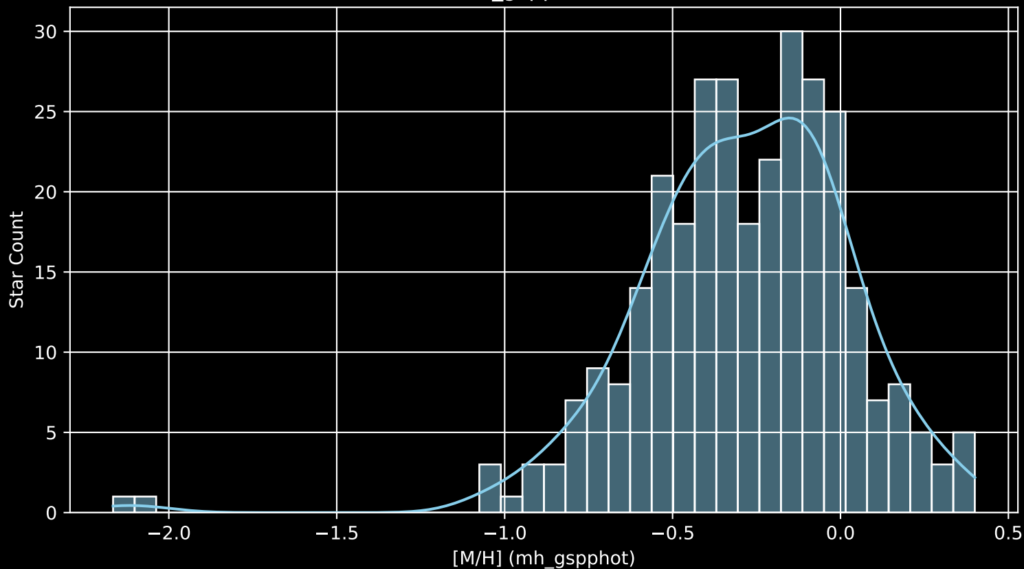
GALAH DR4 Field: [7007] [M/H] (mh_gspphot) (n= 307)
